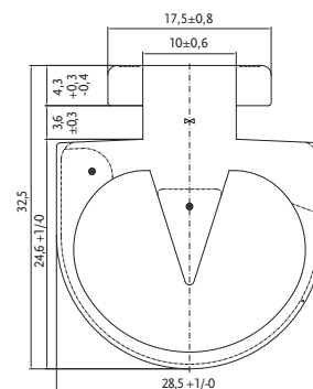
Profilquerschnitt Contact-Duo 3100.0110Y
